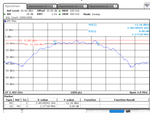
BLE 2Mbps Low
