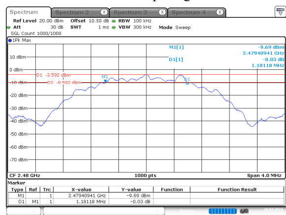
BLE 2Mbps High
