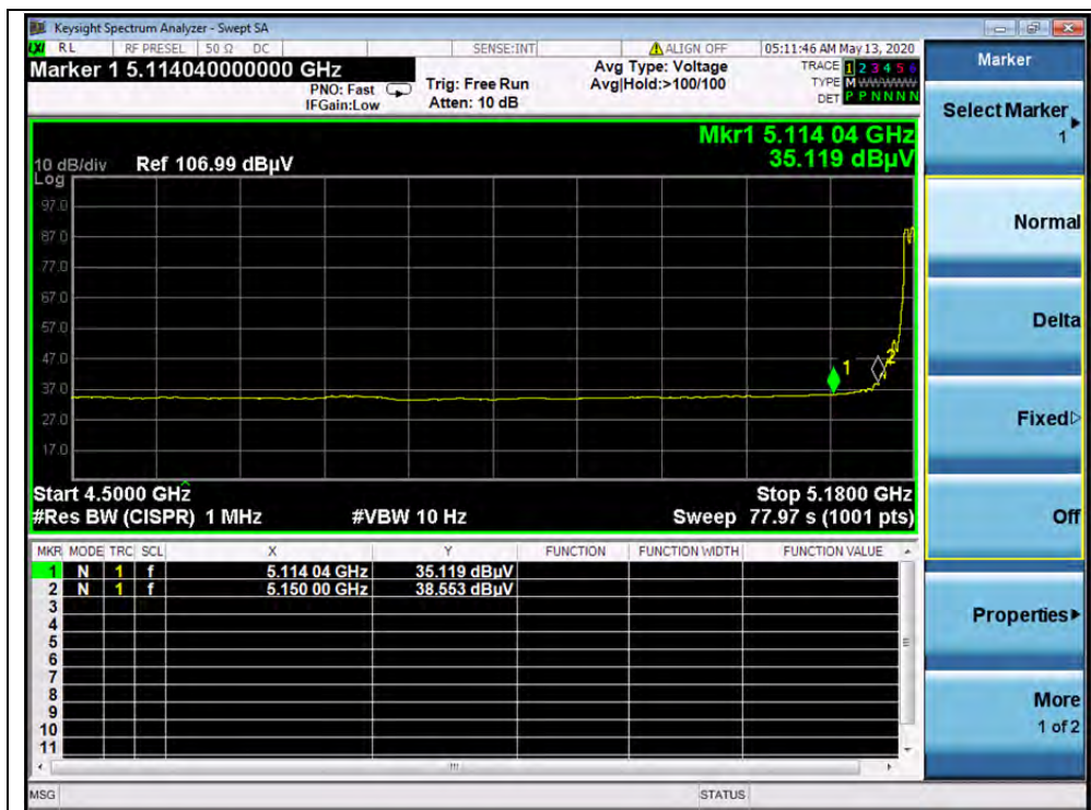
(AVG, Channel 36, 802.11a)
