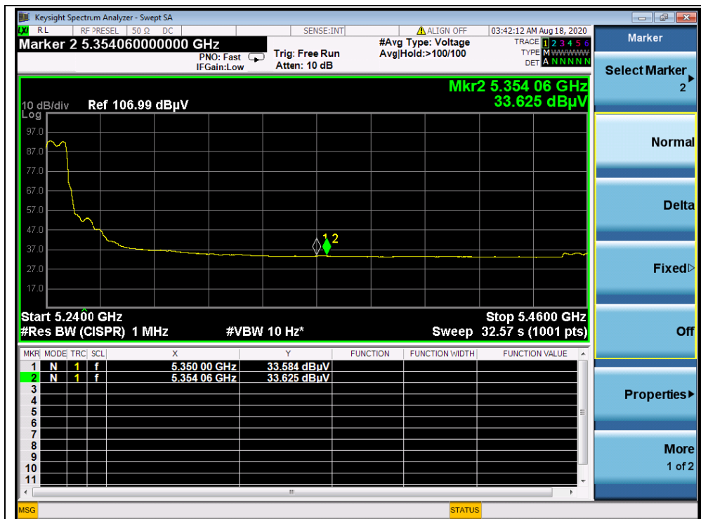
(AVG,Channel 48,802.11a)
