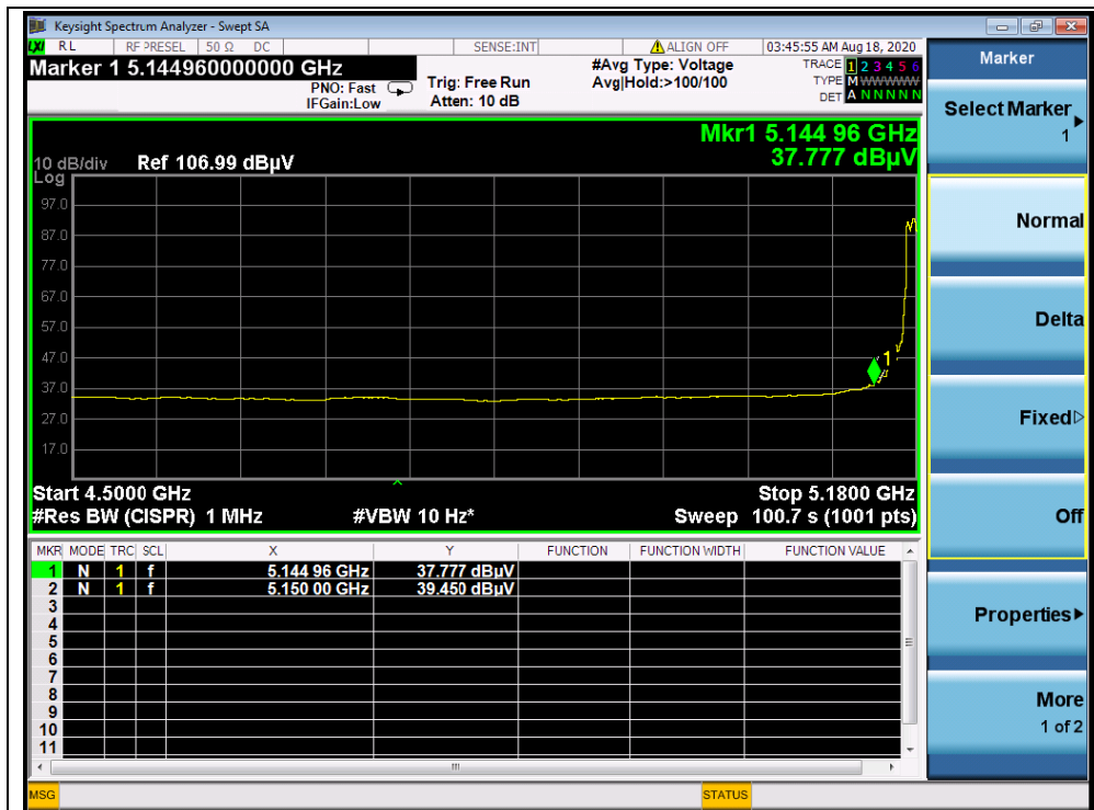
(AVG,Channel 36,802.11a)
