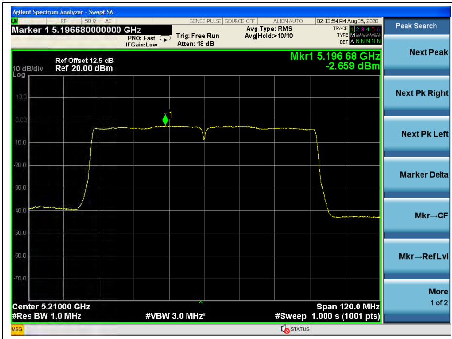
(Channel 42, 5210MHz, 802.11ac (VHT80), ANT L)
