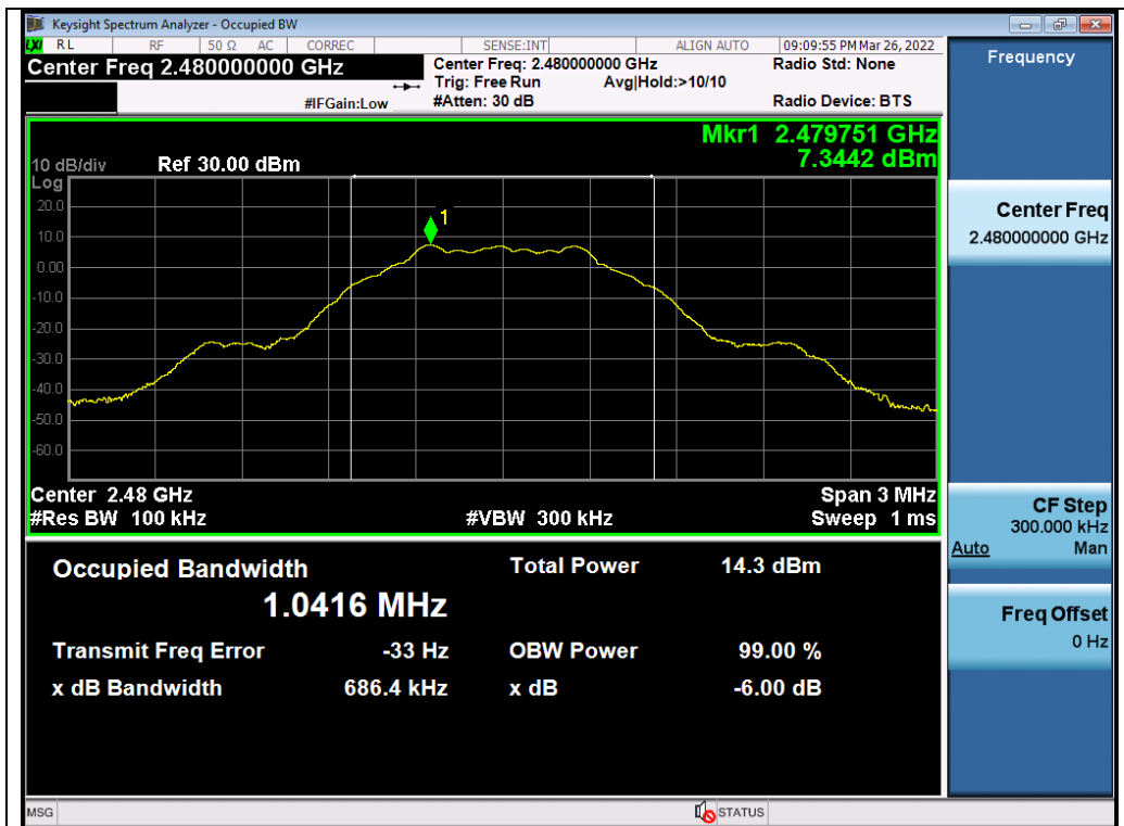
Test_Graph_LE1M_ANT1_2480_1Mbps_DTSSBW
