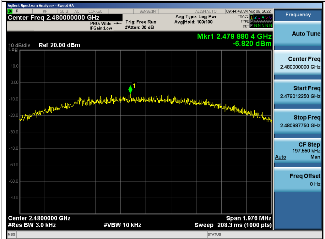
Test_Graph_GFSK_ANT1_2480_2Mbps_PSD
