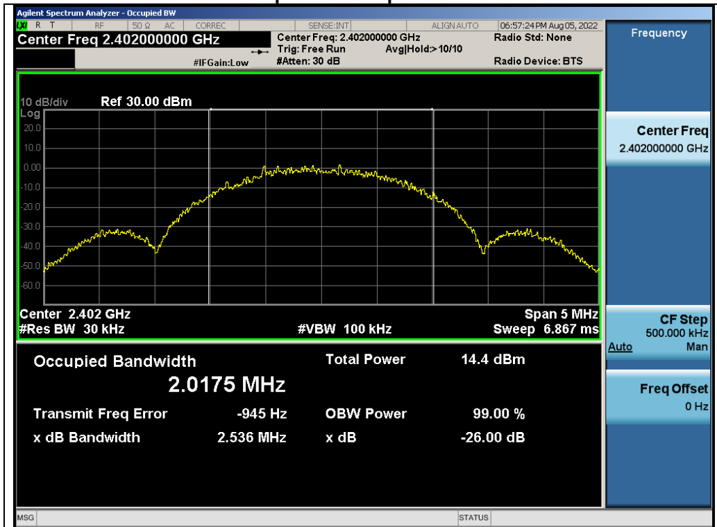
Test_Graph_GFSK_ANT1_2402_2Mbps_OBW
