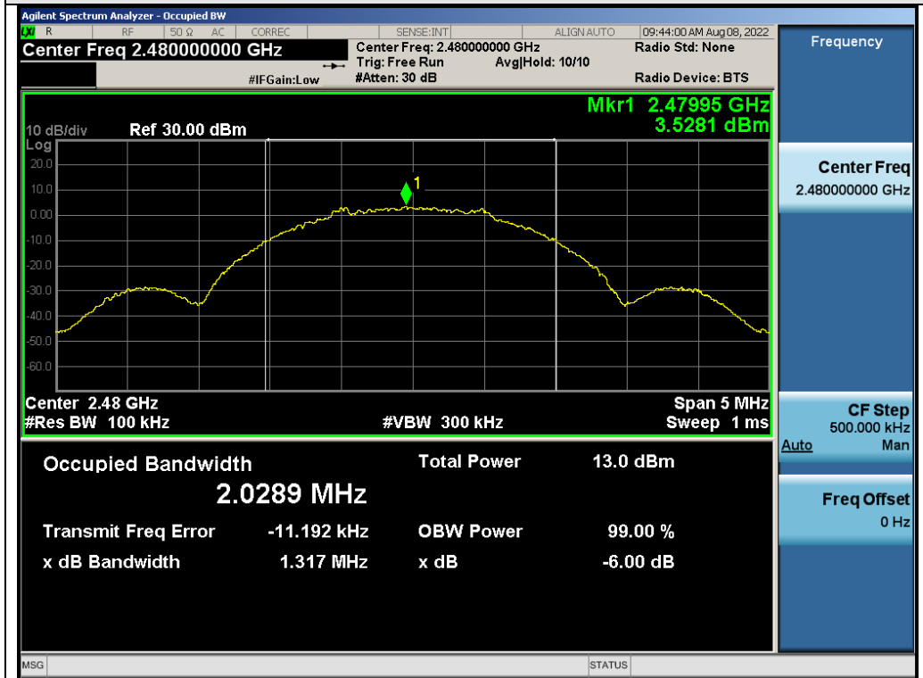
Test_Graph_GFSK_ANT1_2480_2Mbps_DTSSBW
