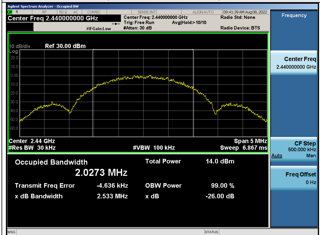
Test_Graph_GFSK_ANT1_2440_2Mbps_OBW
