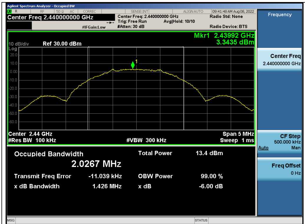
Test_Graph_GFSK_ANT1_2440_2Mbps_DTSSBW
