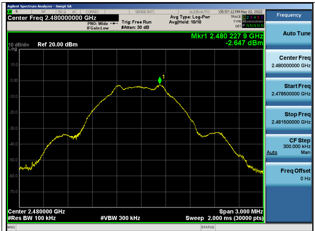
Test_Graph_2.4G_ANT1_2480_Reference Level
