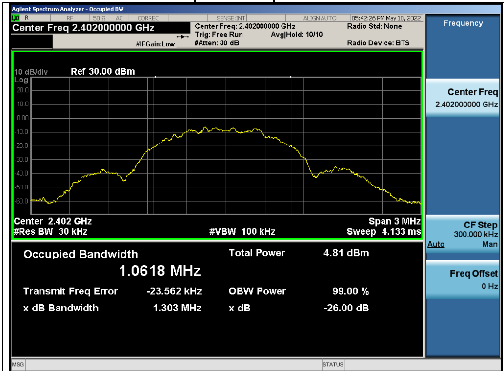
Test_Graph_2.4G_ANT1_2402_OBW
