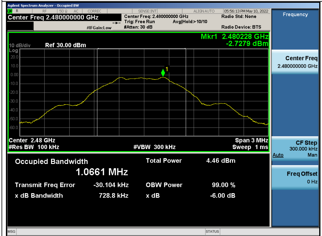
Test_Graph_2.4G_ANT1_2480_DTSBW
