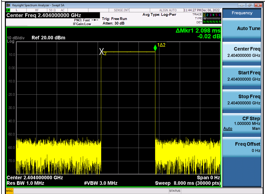
Test_Graph_2.4G_HOP_ANT2_NA_1Mbps_2404_Time per Burst
