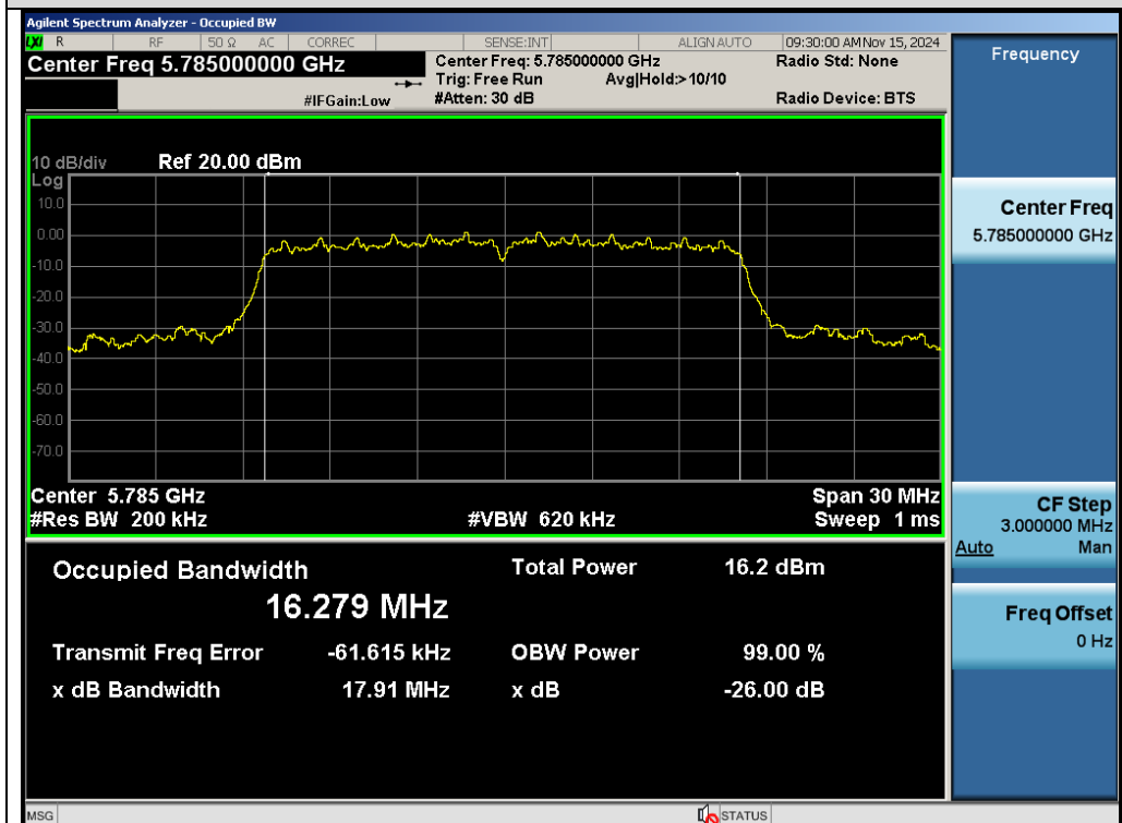
Test_Graph_802.11a_ANT1_5785_6Mbps_OBW
