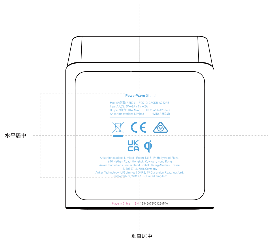
底视图
