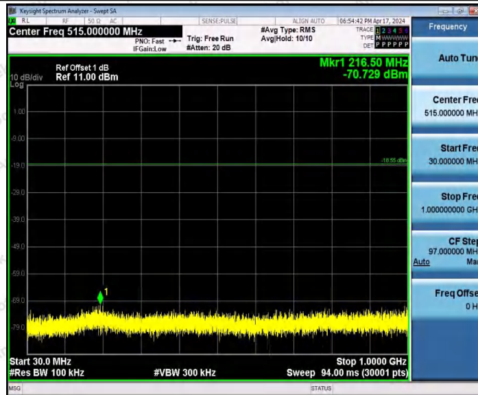
BLE_2M-Ant1-2440-30~1000-PASS
