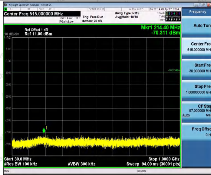
BLE_2M-Ant1-2402-30~1000-PASS
