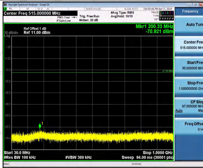
BLE_2M-Ant1-2480-30~1000-PASS
