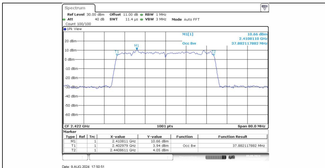
11AX40SISO_Ant1_2422
