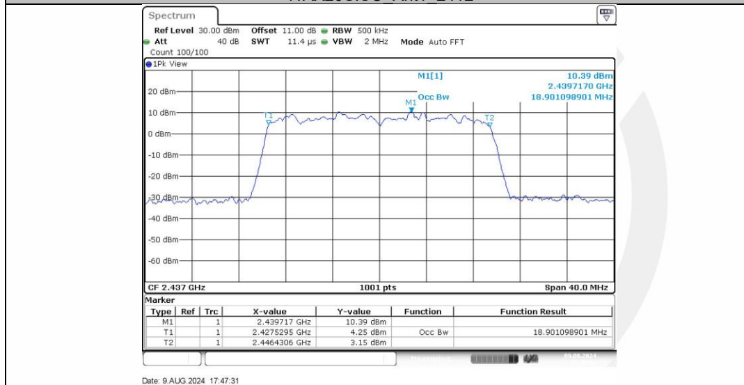
11AX20SISO_Ant1_2437
