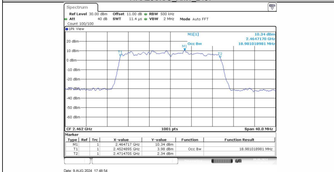
11AX20SISO_Ant1_2462
