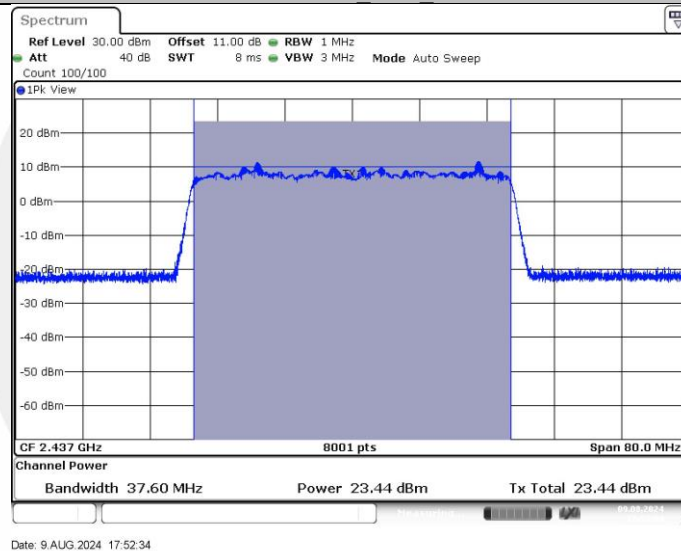
11AX40SISO_Ant1_2437
