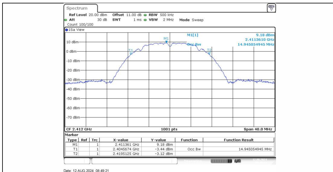
11B_Ant1_2412
