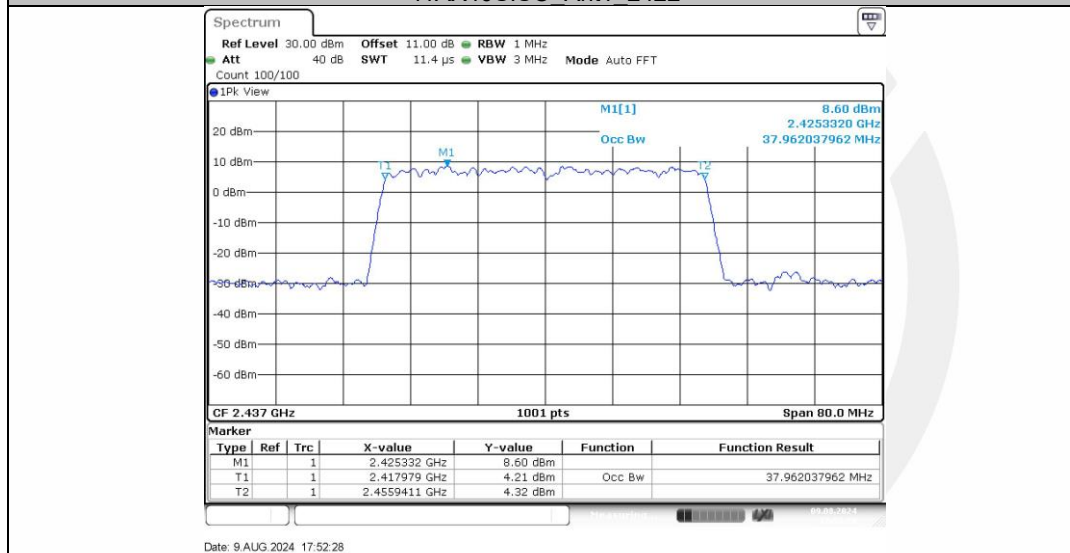
11AX40SISO_Ant1_2437
