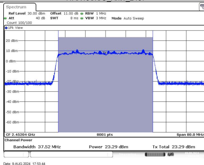
11AX40SISO_Ant1_2452
