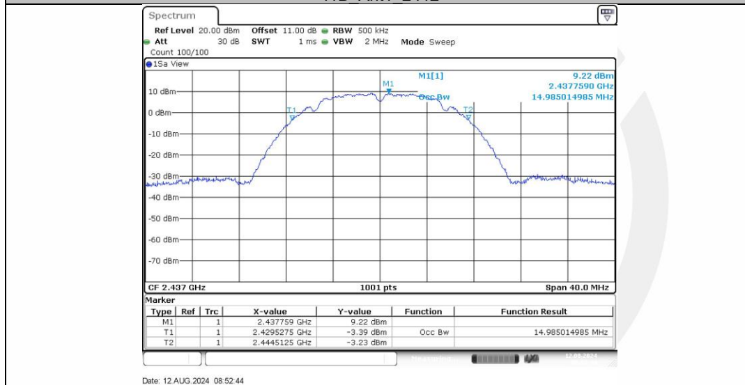
11B_Ant1_2437
