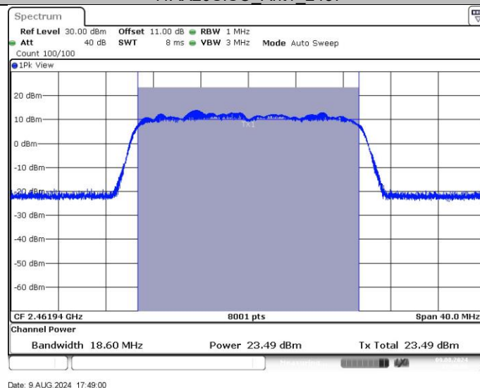
11AX20SISO_Ant1_2462
