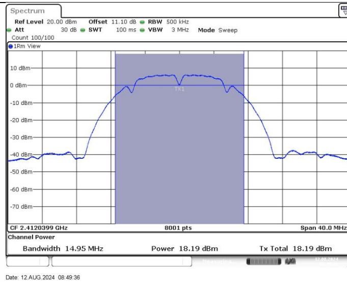
11B_Ant1_2412
