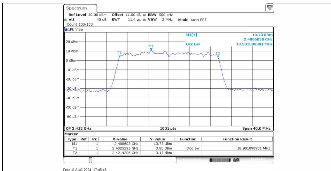
11AX20SISO_Ant1_2412
