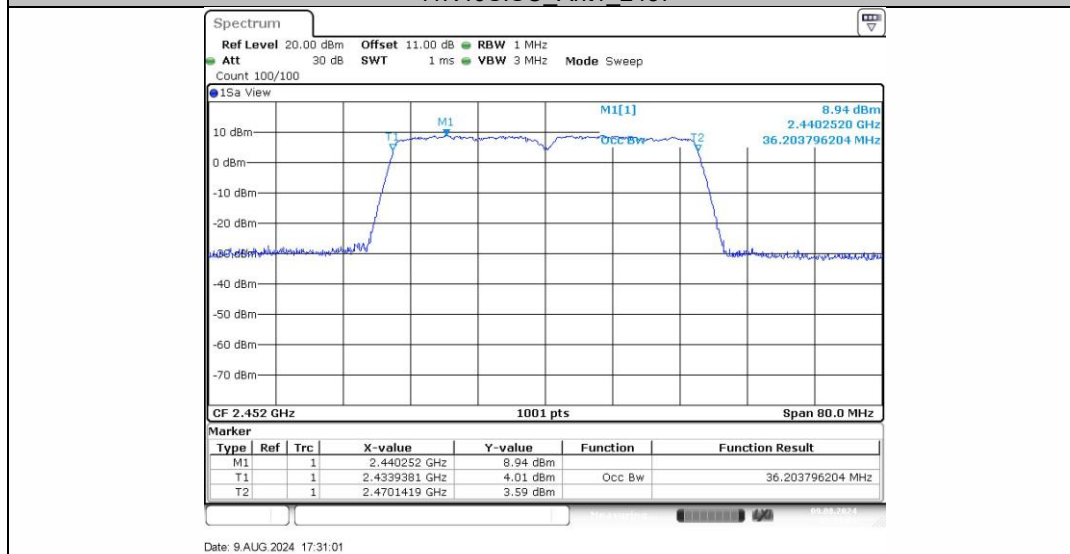
11N40SISO Ant1 2452
