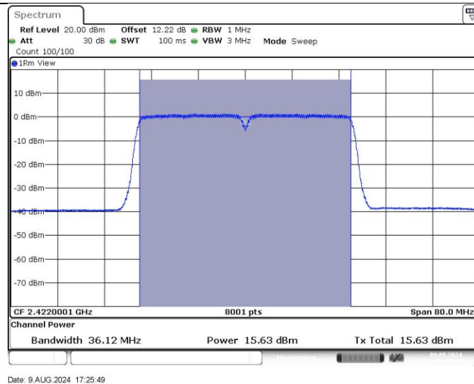
11N40SISO Ant1 2422
