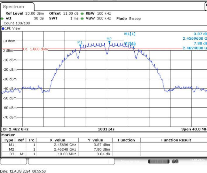
11B_Ant1_2462
