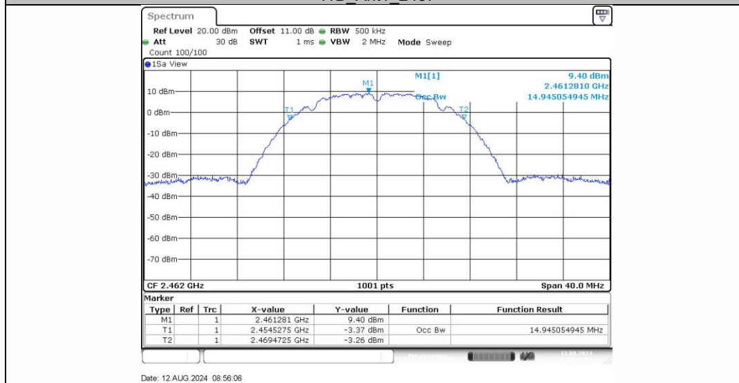
11B_Ant1_2462
