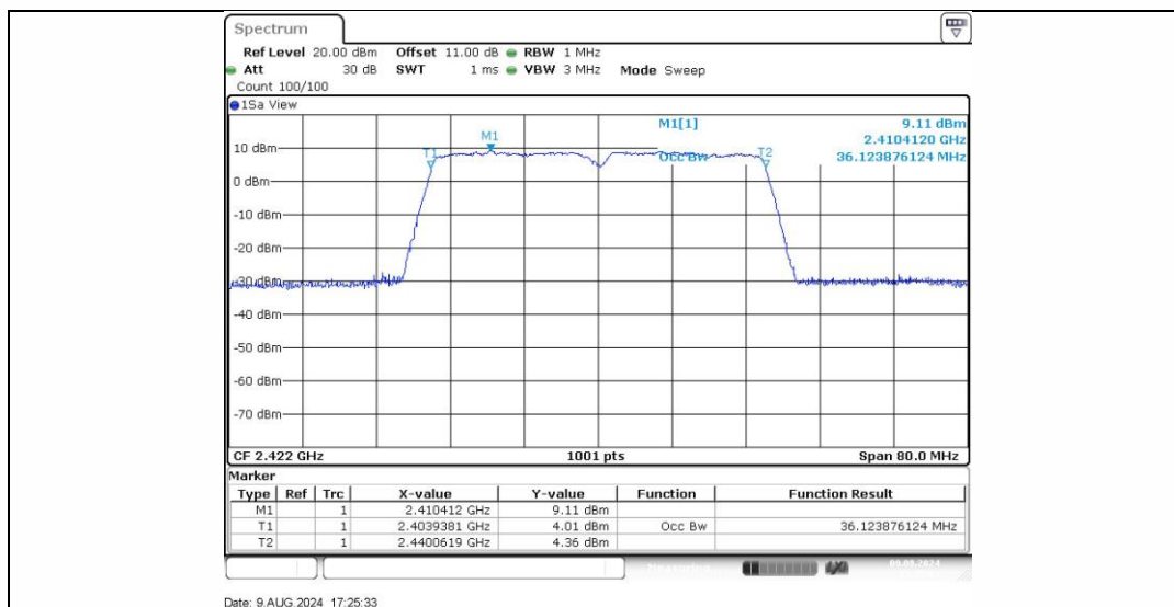
11N40SISO Ant1 2422
