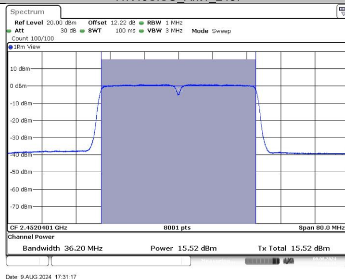
11N40SISO Ant1 2452
