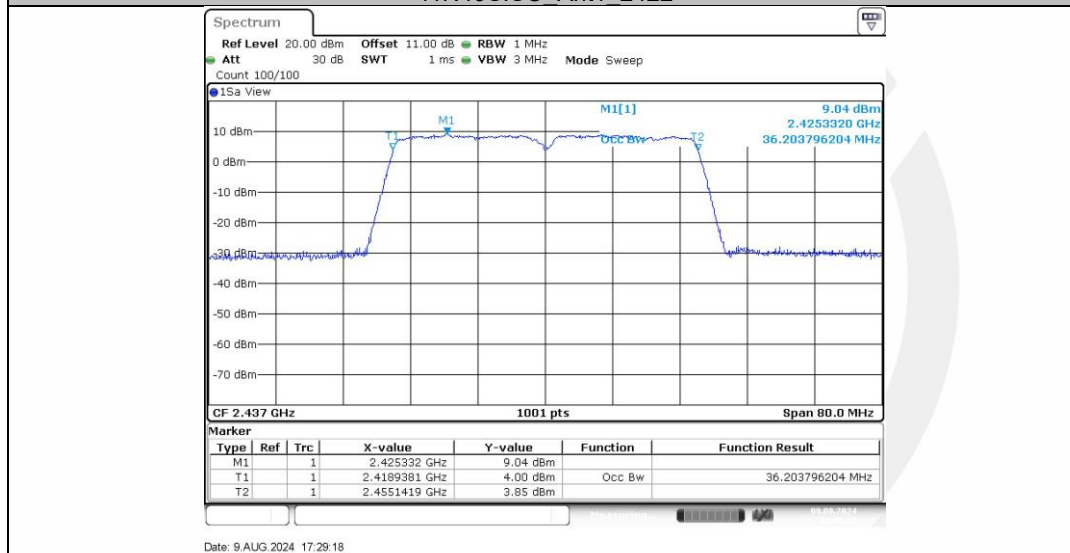
11N40SISO Ant1 2437
