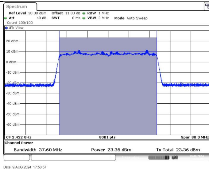
11AX40SISO_Ant1_2422
