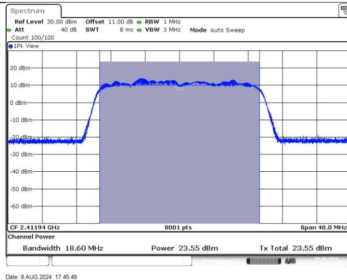
11AX20SISO_Ant1_2412
