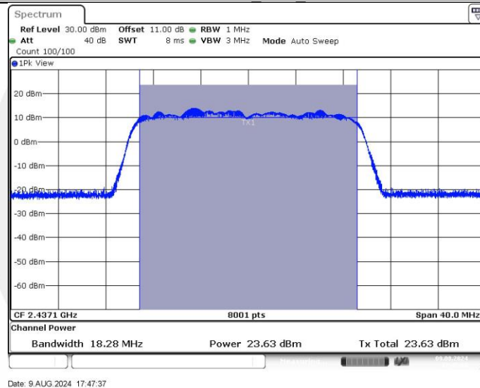
11AX20SISO_Ant1_2437
