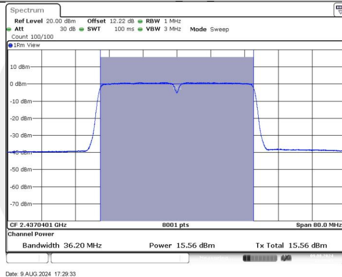
11N40SISO Ant1 2437
