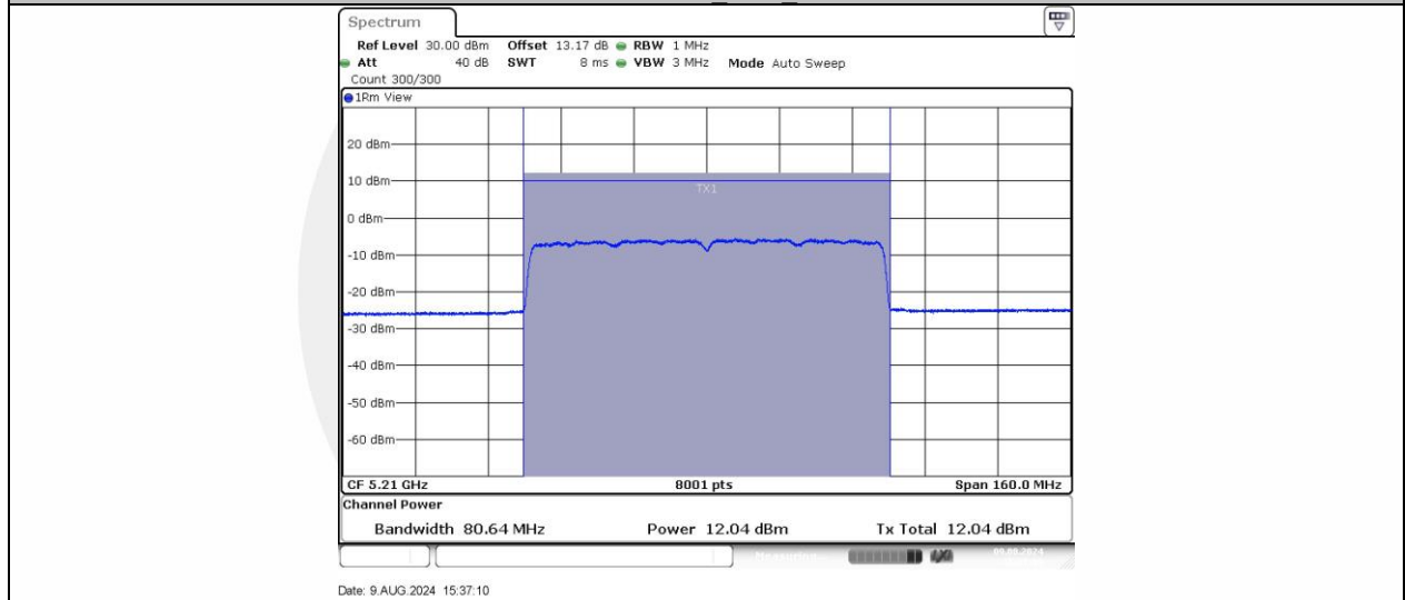
11AX80SISO Ant1 5210
