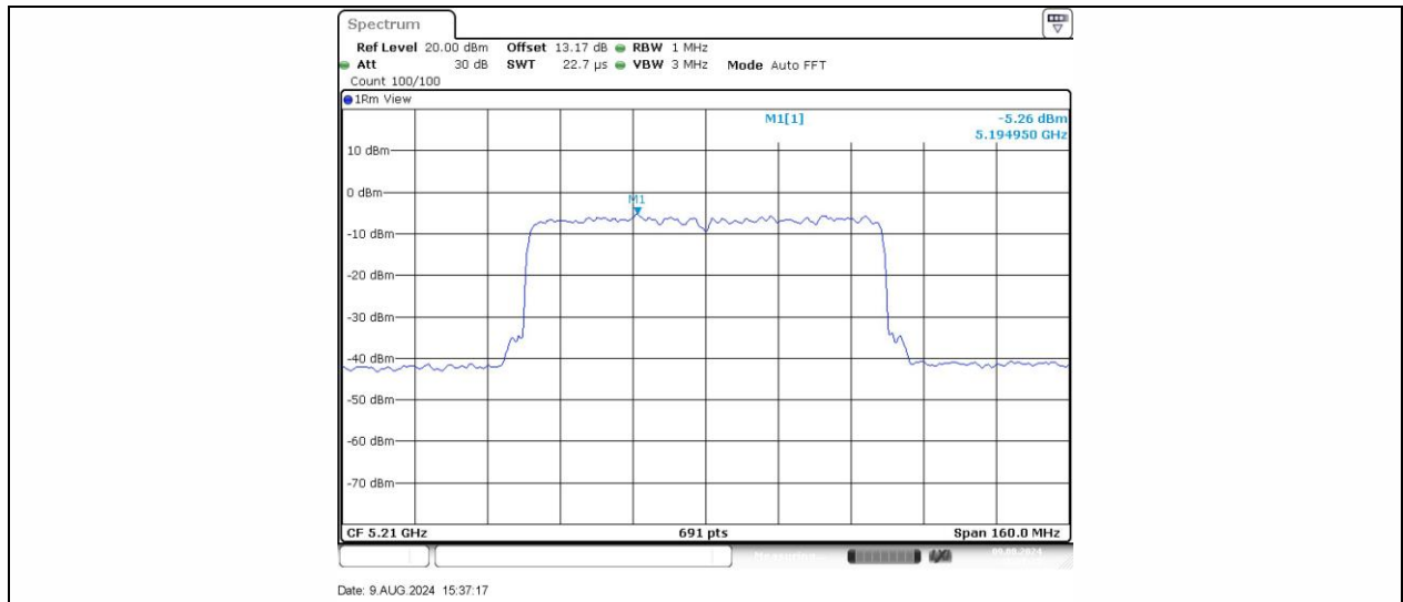
11AX80SISO Ant1 5210
