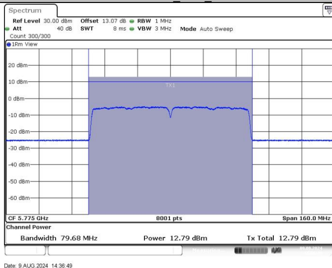
11AC80SISO Ant1 5775
