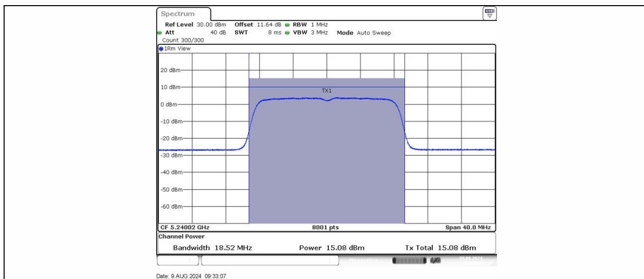
11A Ant1 5240
