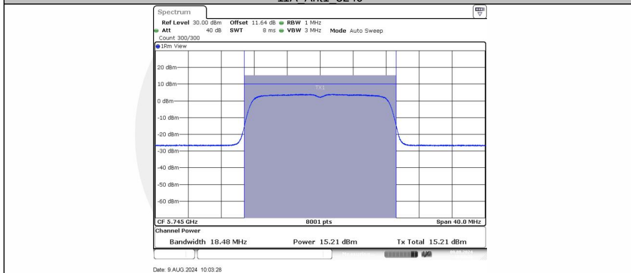
11A Ant1 5745
