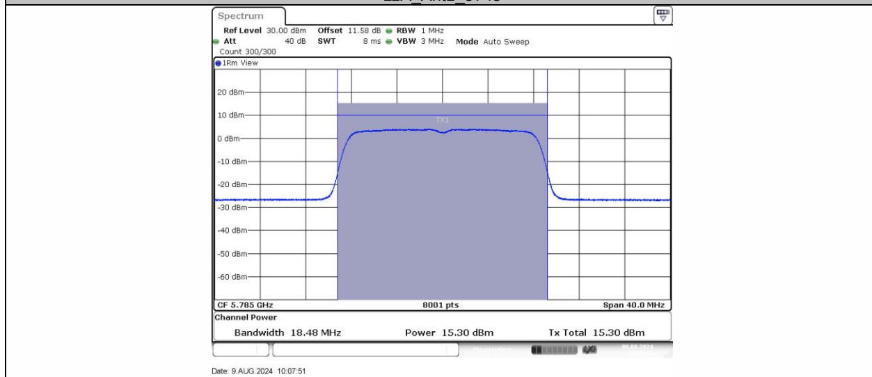
11A Ant1 5785
