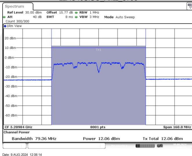
11AC80SISO Ant1 5210
