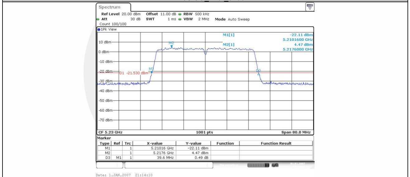
11N40SISO_Ant1_5230
