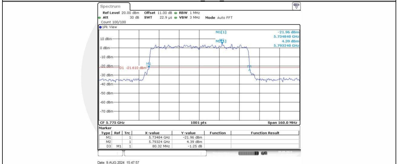
11AX80SISO Ant1 5775
