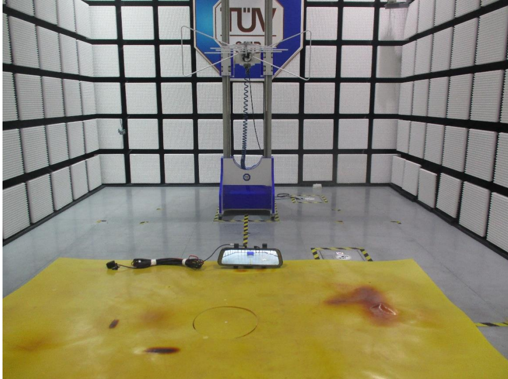
30MHz-1000MHz RSE Setup
