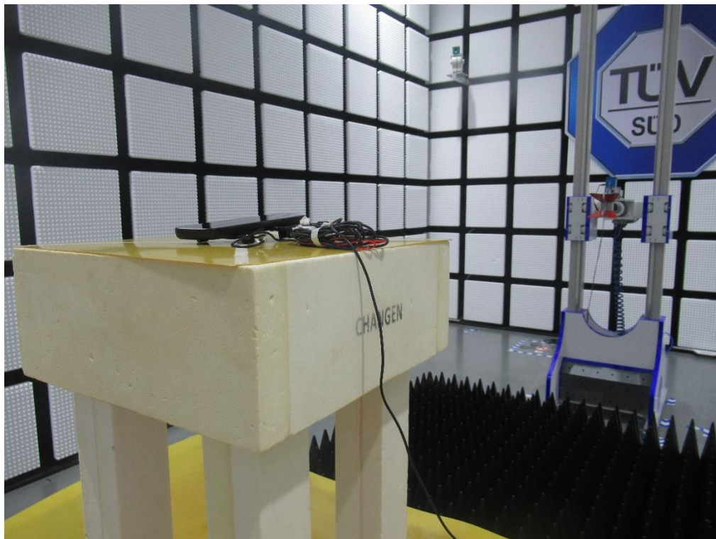
1GHz-18GHz RSE Setup
