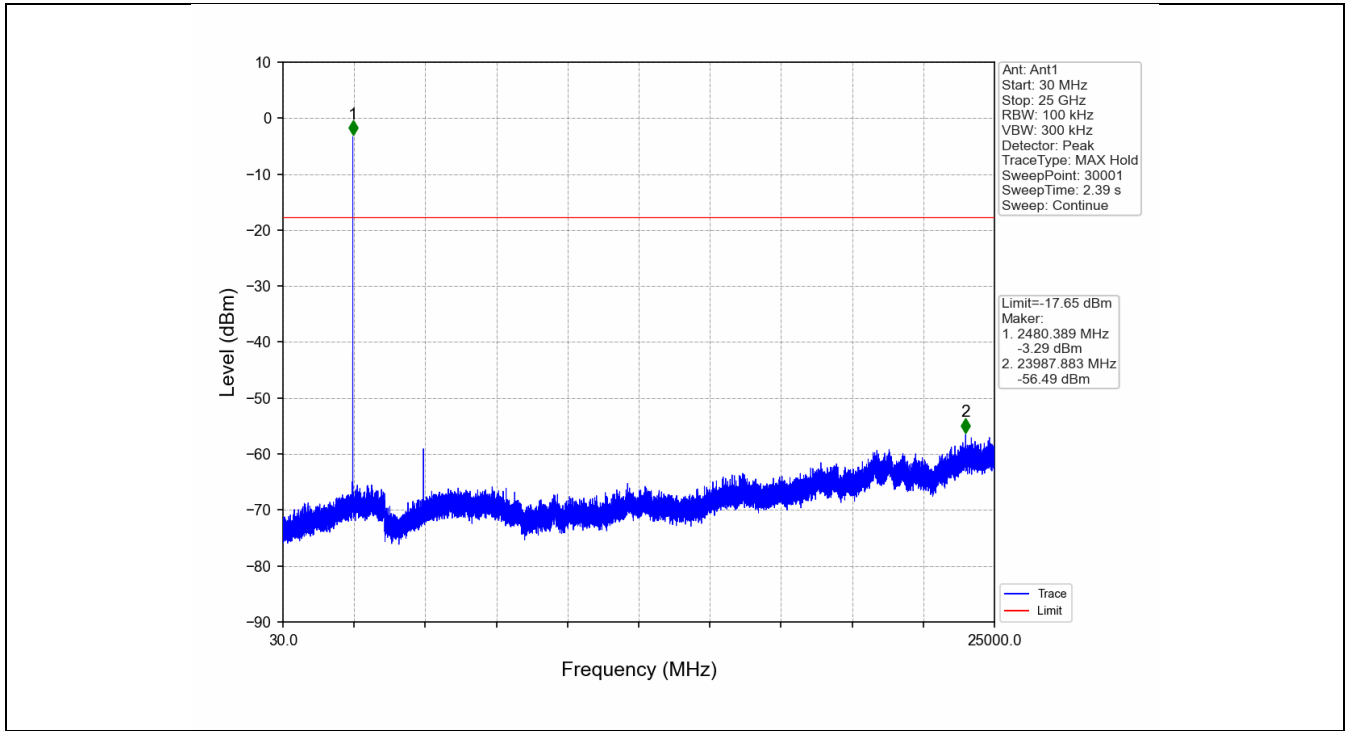
Pi/4DQPSK_2DH5_HOPP_Ant1_NTNV
