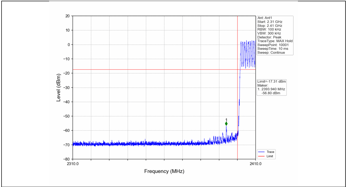
GFSK_DH5_HOPP_Ant1_NTNV
