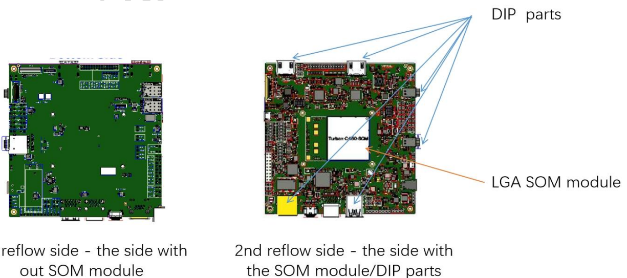
Figure 1-3. SOM Overview
