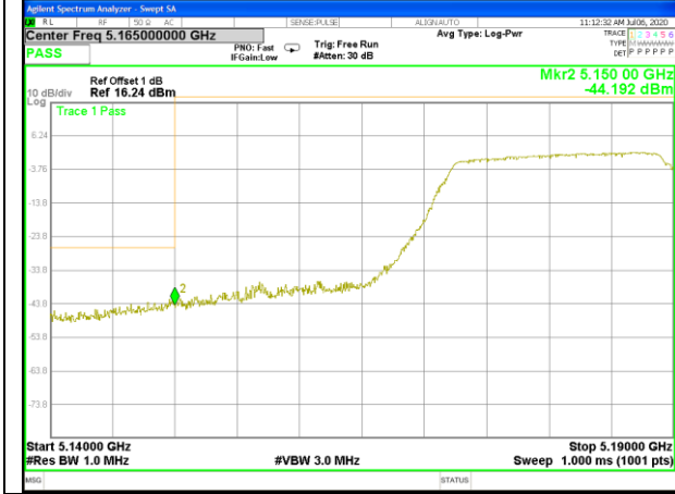
W52_11n40_Lower_Band edge
