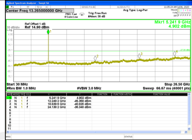
W52_11n20_Higher_Band edge
