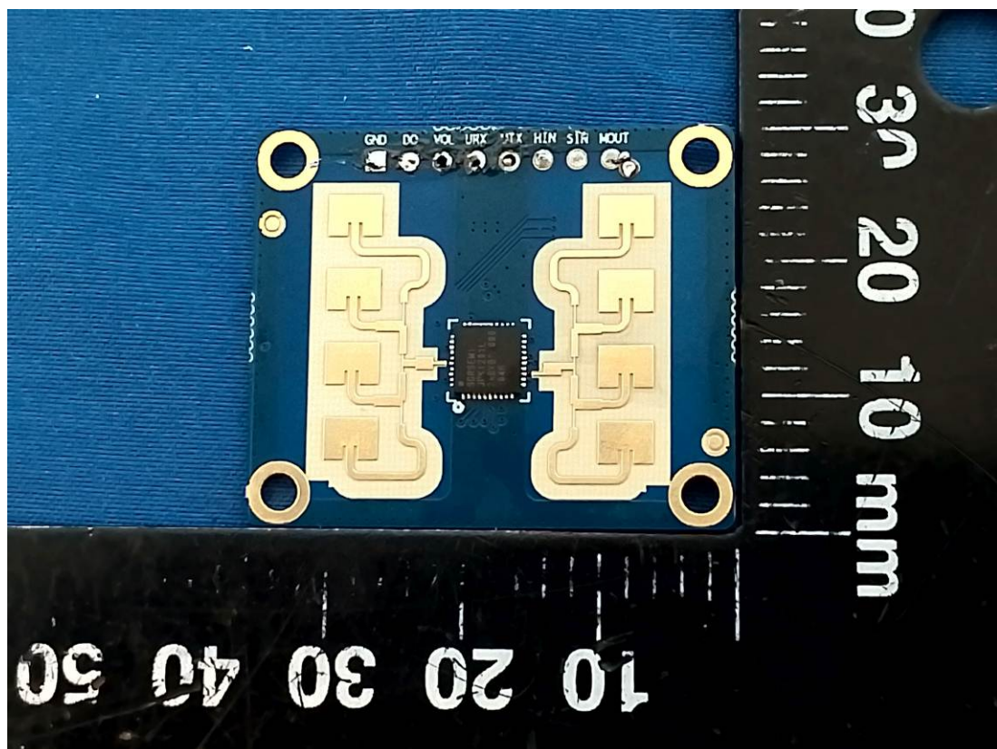
Radar Module
