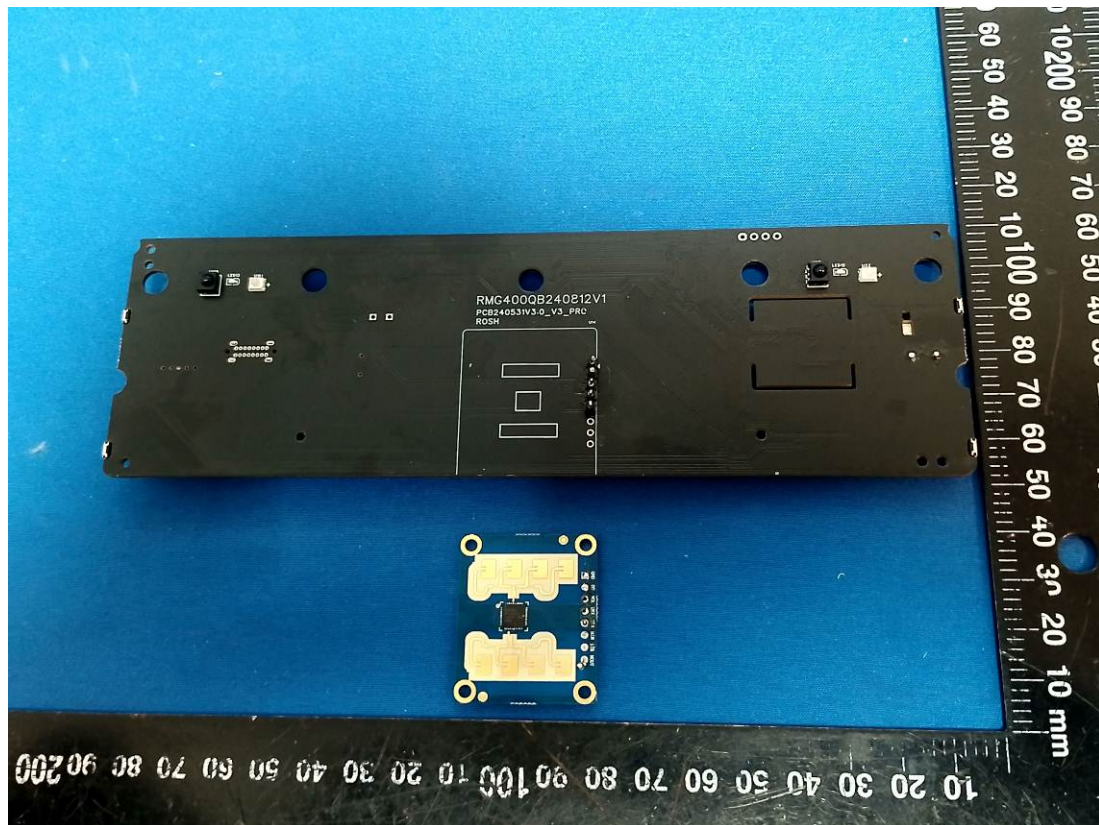
Radar Module
