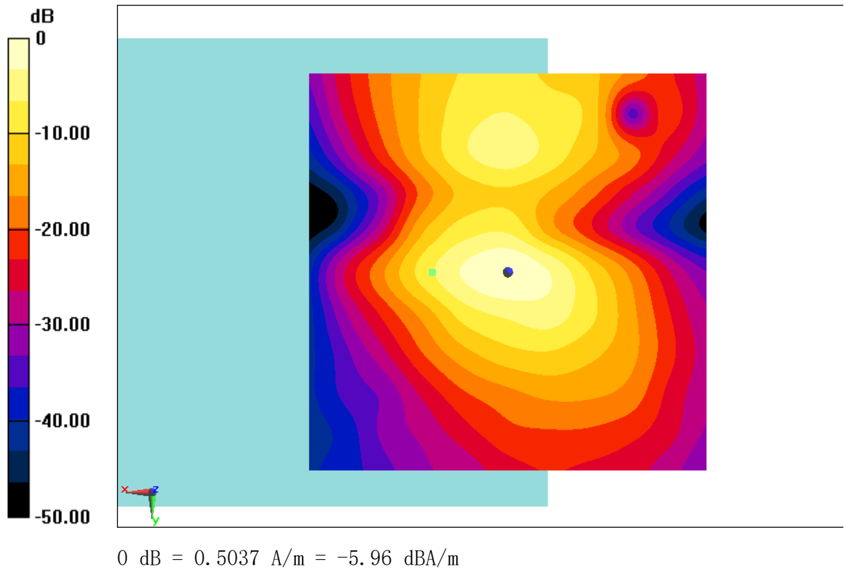
Fig B.21 T-Coil WiFi-2. 4G
