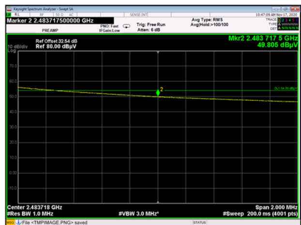
O-QPSK (Zigbee) CH26, AV
