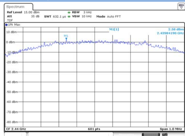
GFSK (BLE) CH19
