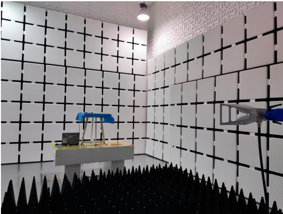
RSE 1GHz-18GHz
