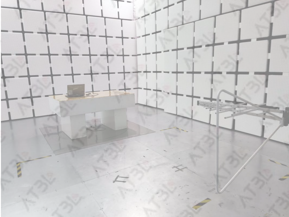
RSE 30MHz-1000MHz
