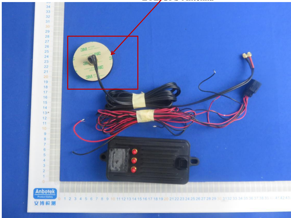
LTE/GPS Antenna
