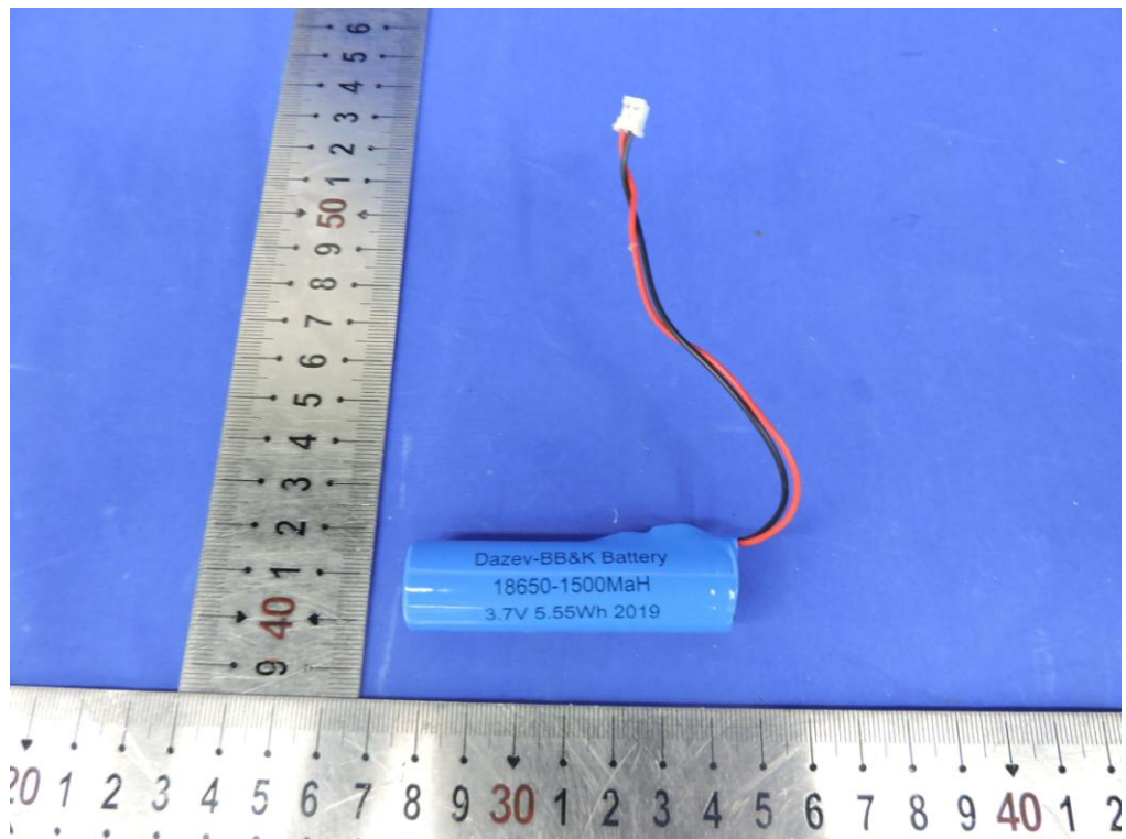
EUT Photo 6
