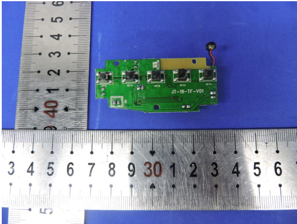
EUT Photo 3
