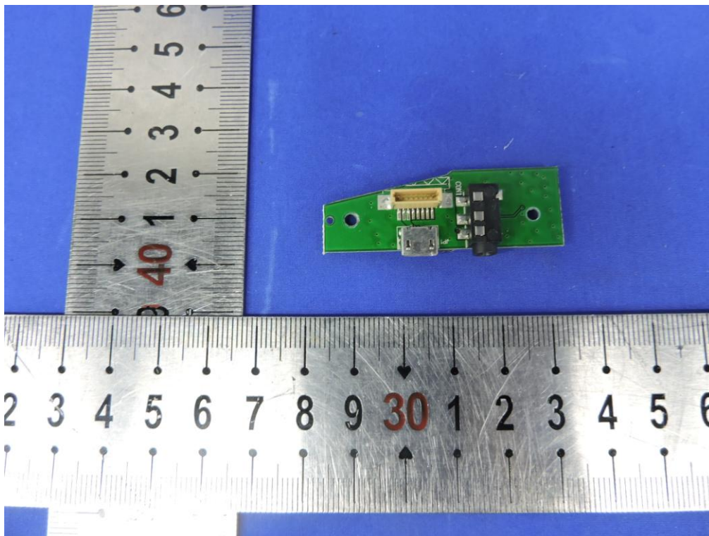
EUT Photo 4
