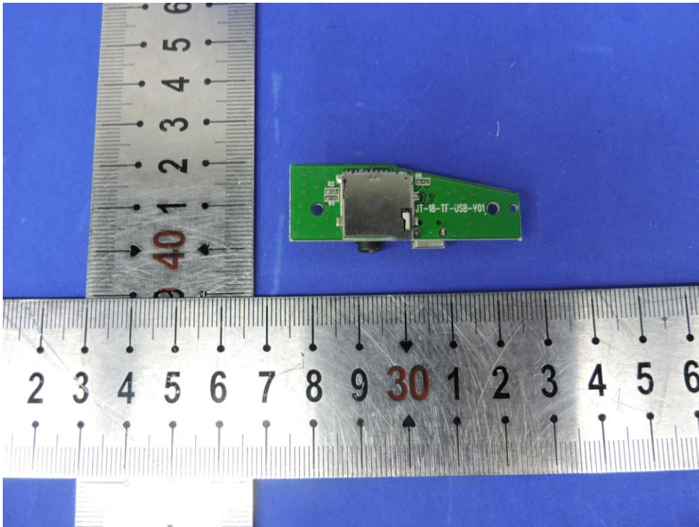
EUT Photo 5
