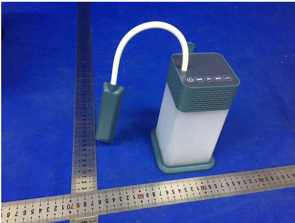
EUT Photo 2
