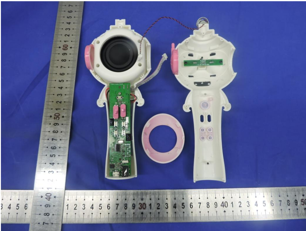
EUT Photo 1
