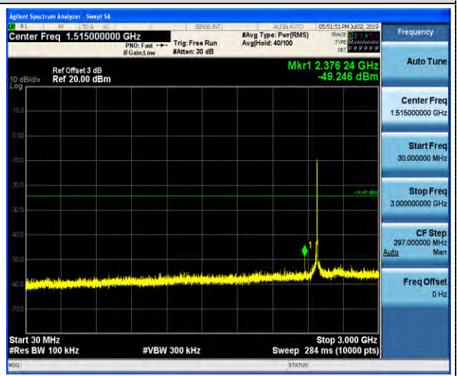
30MHz-3GHz
