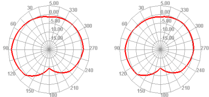
Bluetooth 39 TRP E1
