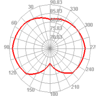
Bluetooth 39 TIS E1
