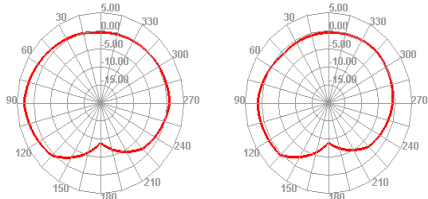
Bluetooth 78 TRP E1
