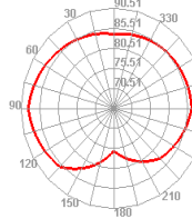
Bluetooth 39 TIS E1
