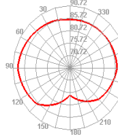
Bluetooth 78 TIS E1
