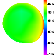
Bluetooth 78 TIS E1
