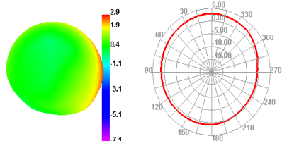
Bluetooth 78 TRP E1
