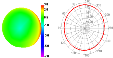
Bluetooth 39 TRP E1
