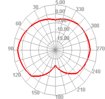
Bluetooth 39 TRP E2
