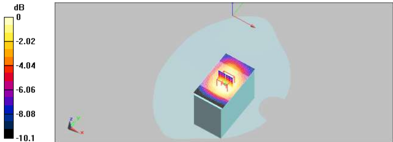
0 dB = 0.188mW/g
