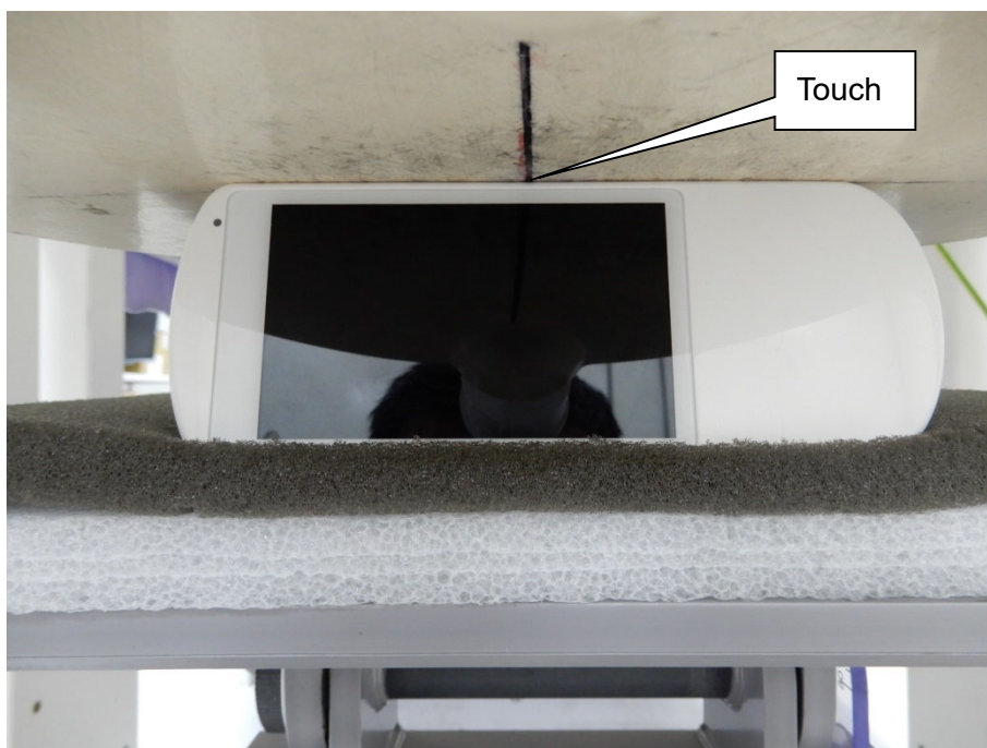
EUT Right-side
