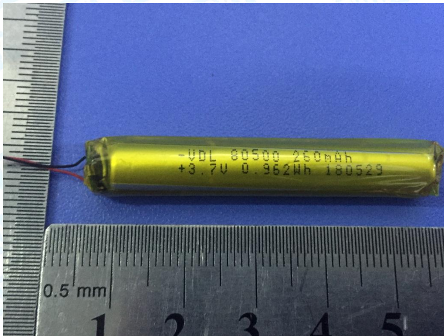
Photo 12 Battery Parameter
