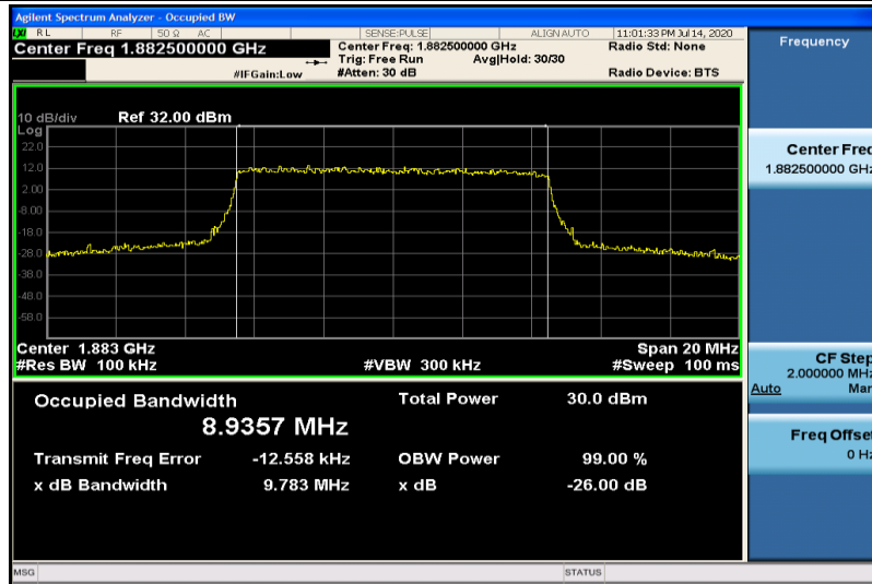
Band25-10MHz-QPSK-26365-50RB#0-8.9357
