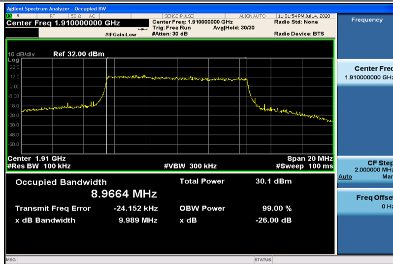
Band25-10MHz-QPSK-26640-50RB#0-8.9664
