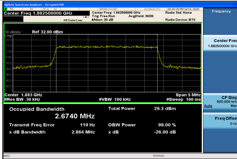
Band25-3MHz-QPSK-26365-15RB#0-2.6740
