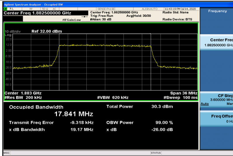
Band25-20MHz-QPSK-26365-100RB#0-17.841
