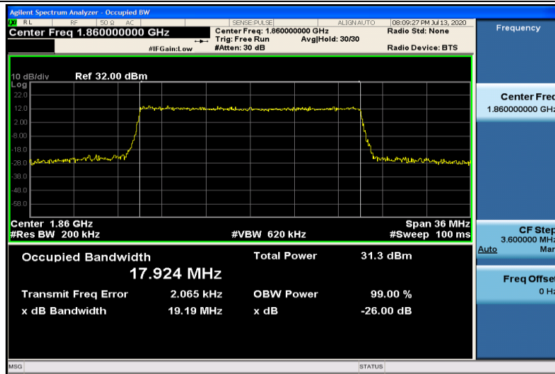
Band2-20MHz-QPSK-18700-100RB#0-17.924
