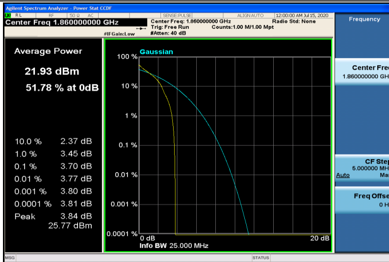
Band25-20MHz-QPSK-26140-1RB#0
