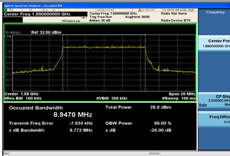
Band2-10MHz-QPSK-18900-50RB#0-8.9470
