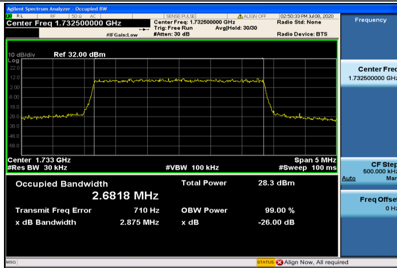
Band4-3MHz-QPSK-20175-15RB#0-2.6818
