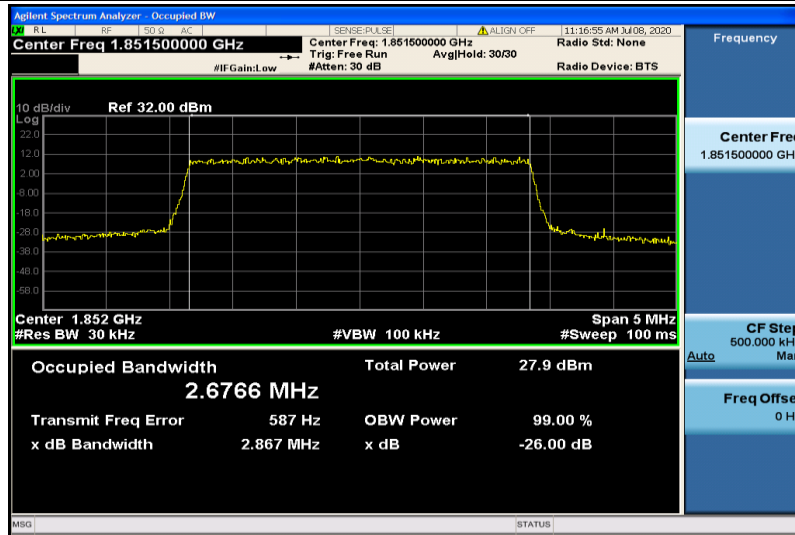
Band2-3MHz-QPSK-18615-15RB#0-2.6766
