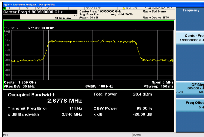
Band2-3MHz-QPSK-19185-15RB#0-2.6776
