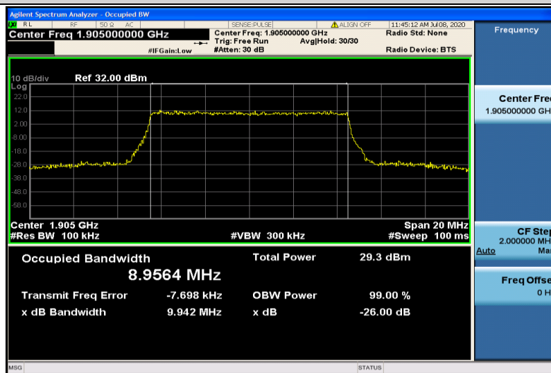
Band2-10MHz-QPSK-19150-50RB#0-8.9564
