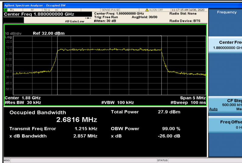
Band2-3MHz-QPSK-18900-15RB#0-2.6816
