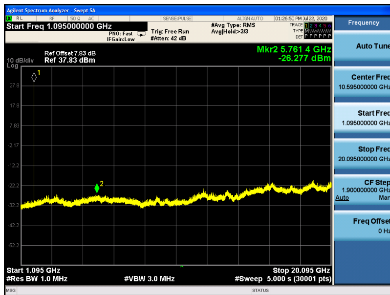
GPRS1900-810-1000~20000
