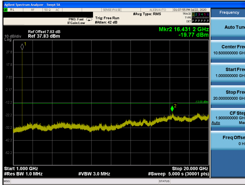
GSM1900-661-1000~20000
