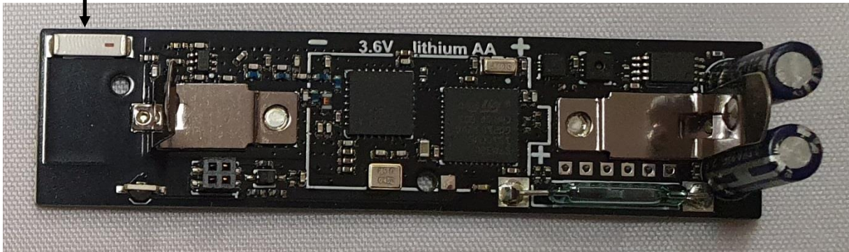
PCB-top
