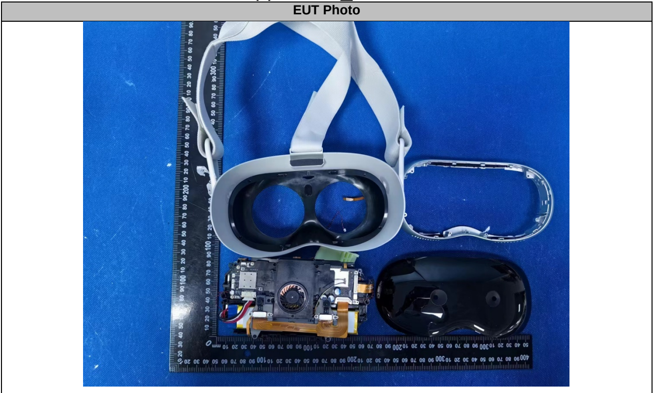
EUT Photo
