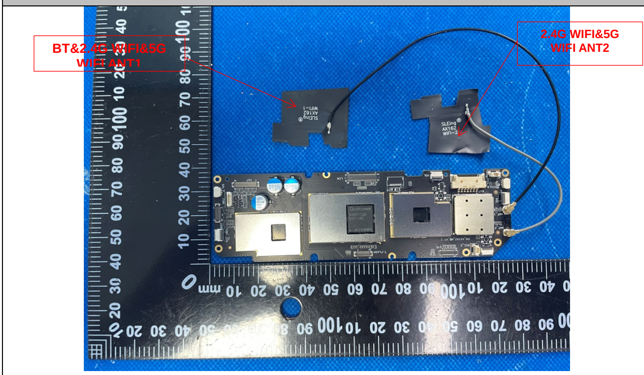
EUT Photo
