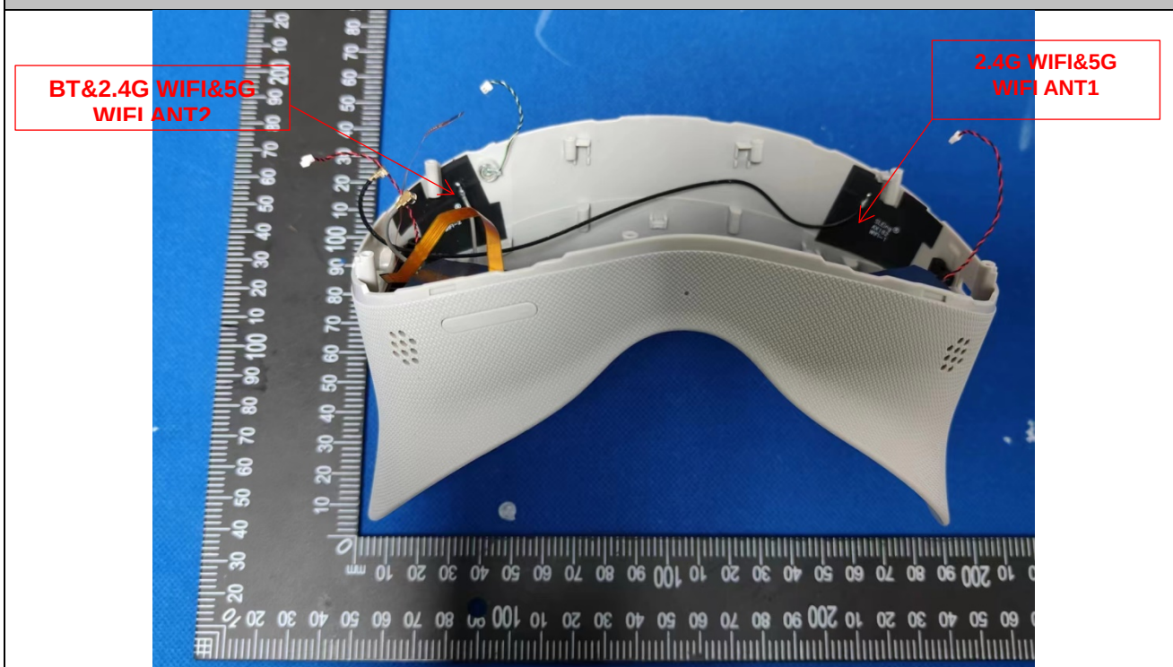
EUT Photo
