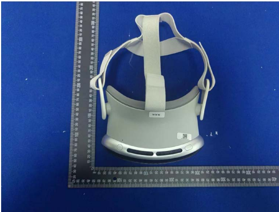
EUT Photo
