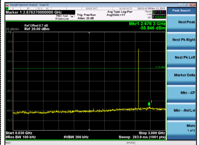
30MHz-3GHz
