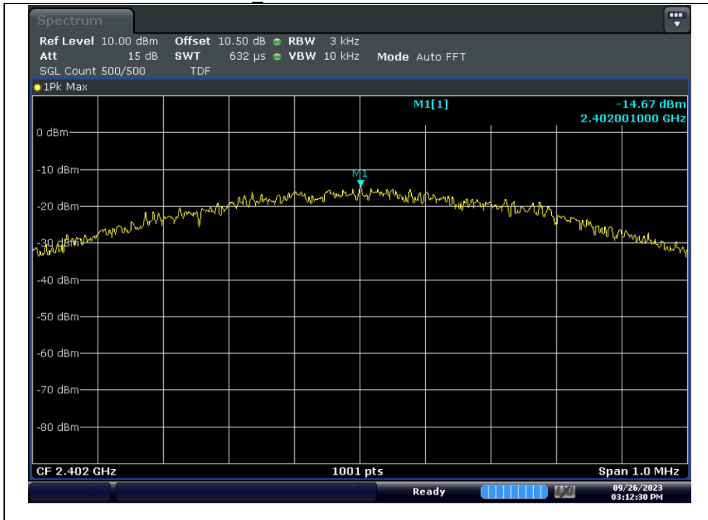
Test mode : Bluetooth LE 1M 2 402 MHz
