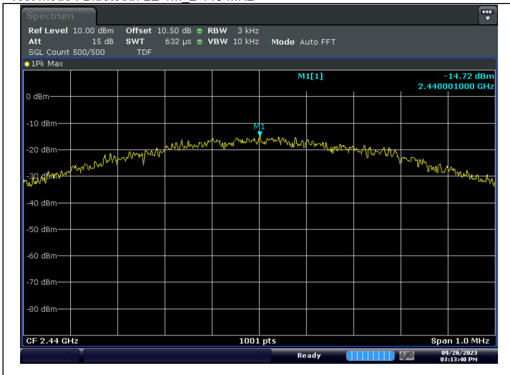
Test mode : Bluetooth LE 1M 2 440 MHz
