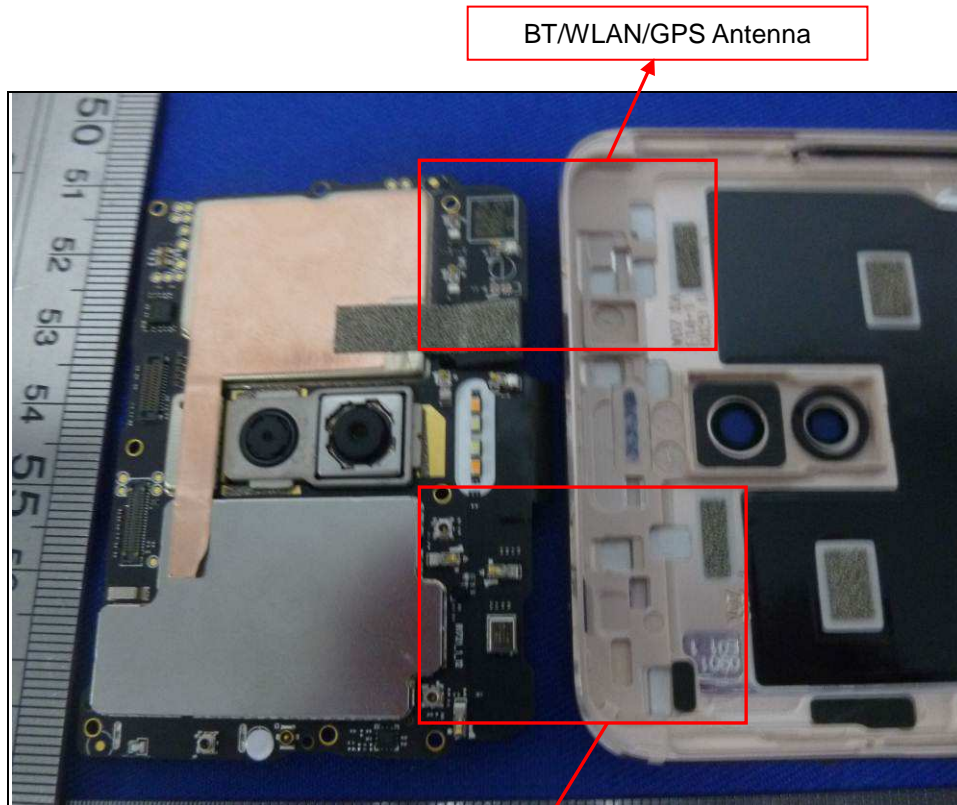
WWAN MIMO Antenna
