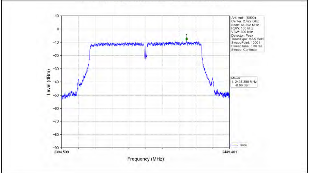
802.11n(HT40)_LCH_2422MHz_Ant1 (SISO)_NTNV
