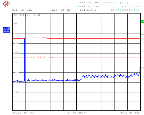
30MHz~25GHz
