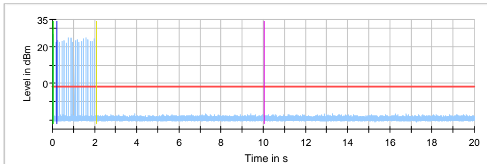
802.11a 5260 MHz_Ant 0+1
