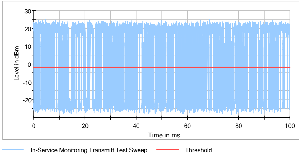
802.11a 5260 MHz_Ant 0+1
