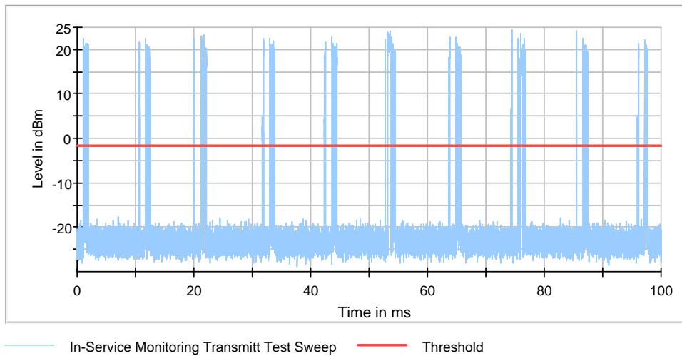
802.11n HT20 5260MHz_Ant 2
