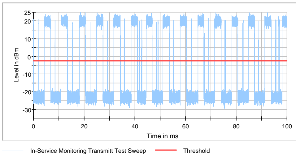
802.11n HT20 5260MHz_Ant 0+1
