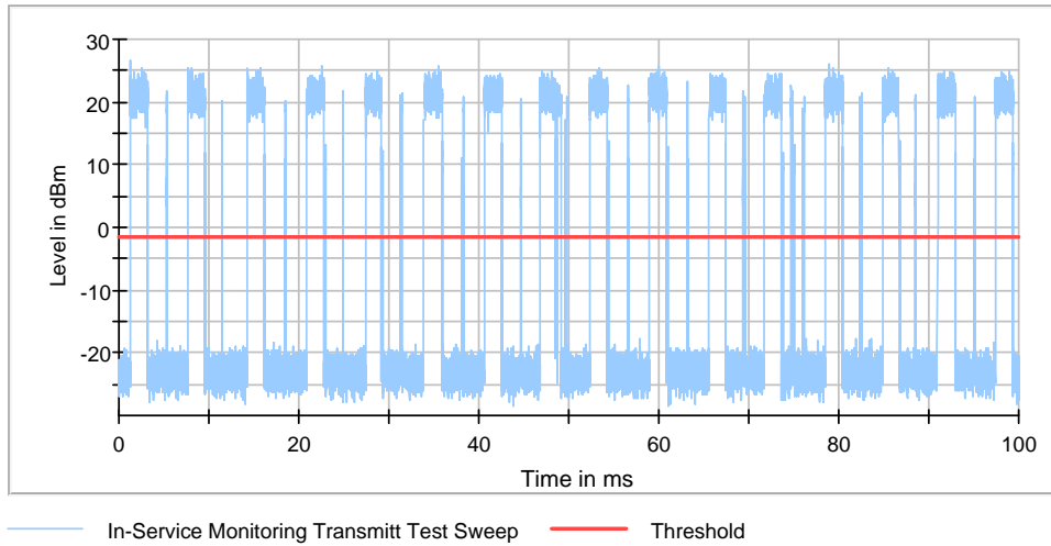
802.11ac VHT20 5260MHz_Ant 0+1
