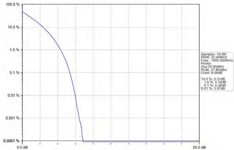
Band25_20MHz_QPSK_HCH_1905MHz_RB_100_0_NTNV
