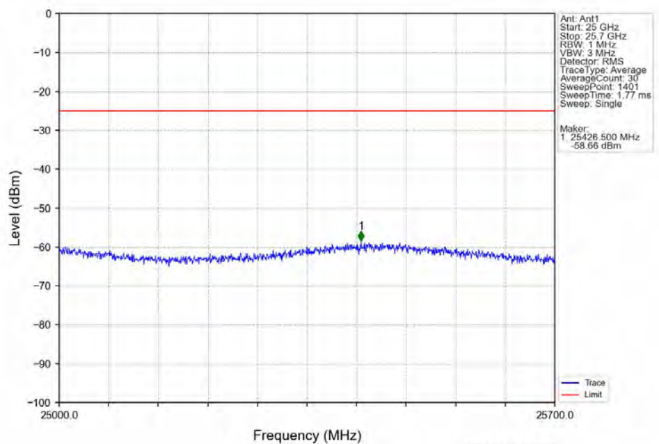
Band7_5MHz_QPSK_LCH_2502.5MHz_RB_1_0_NTNV
