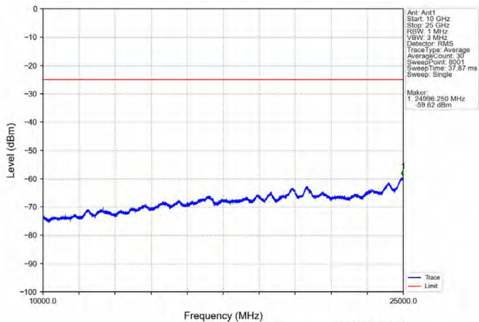
Band7_20MHz_16QAM_LCH_2510MHz_RB_1_0_NTNV
