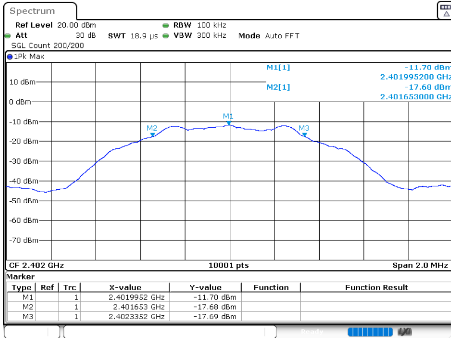
-6 dB BW NVNT BLE 2402MHz 1Mbps
