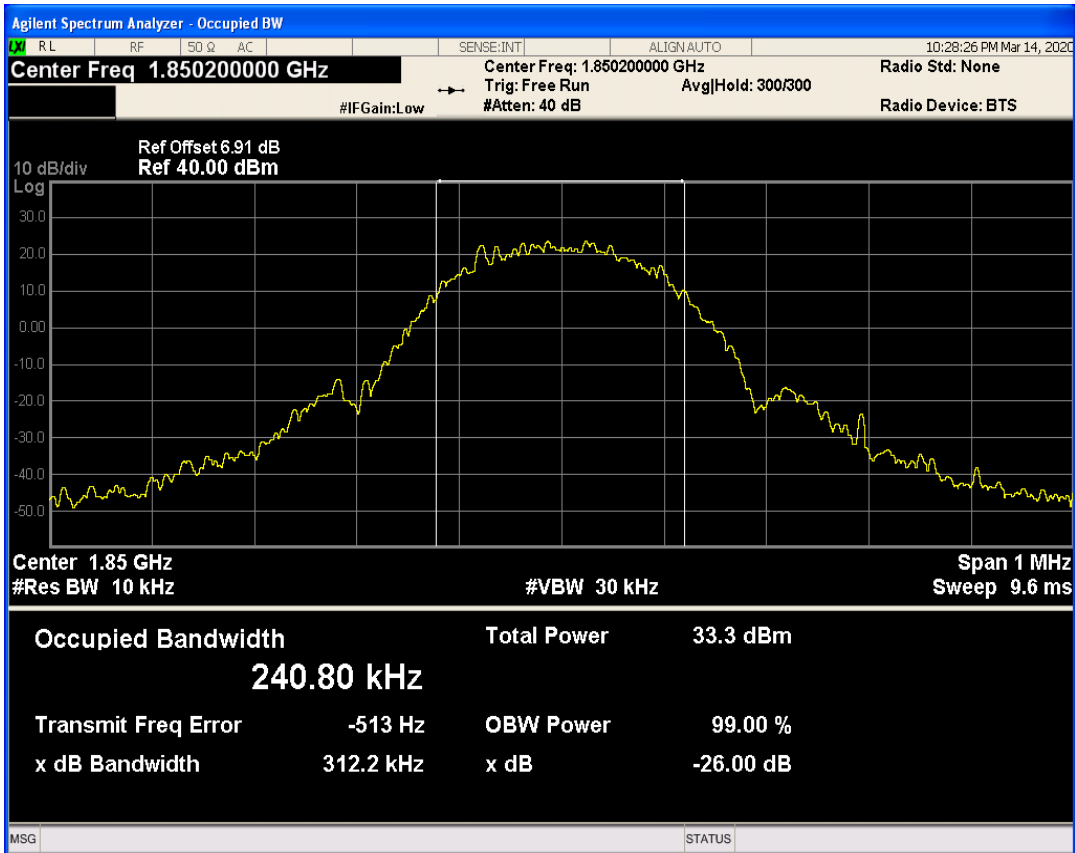
EGPRS1900 Channel=810
