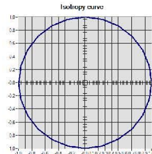
Isotropy +/- 0.21% (+/- 0.01dB)
